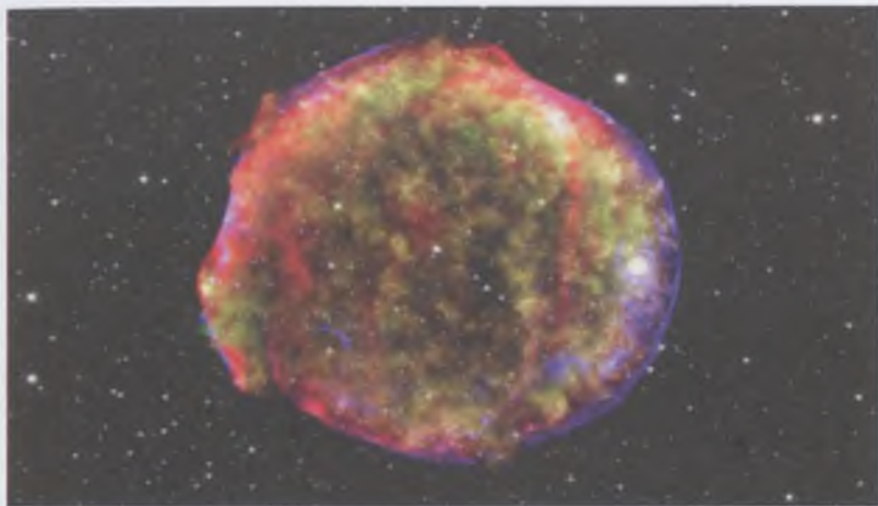
Az 1572-es Tycho Brahe-féle szupernóva maradványa röntgen (Chandra), infravörös (Spitzer) és optikai (Caral Alto Obszervatórium) tartományban készült képek kompozíciójaként. Ez is egy Ia típusú robbanás volt
