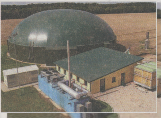
97. ábra. Biogáz-energiatermelő berendezés (Kijev megye)
